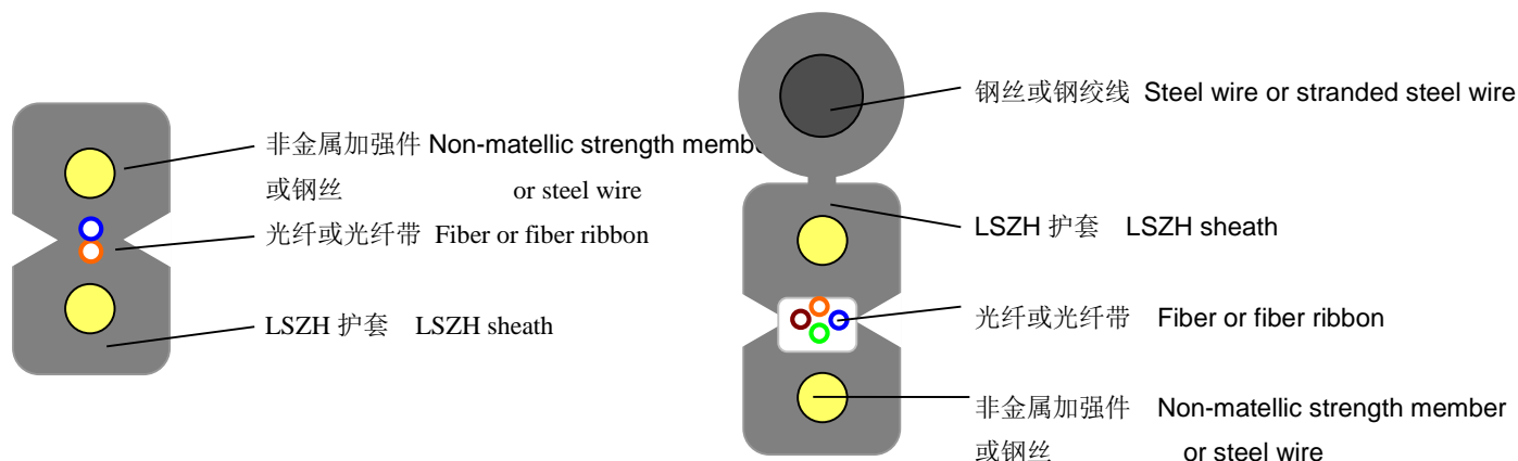
图一 Figure 1 产品技术参数/ Technical parameter:
